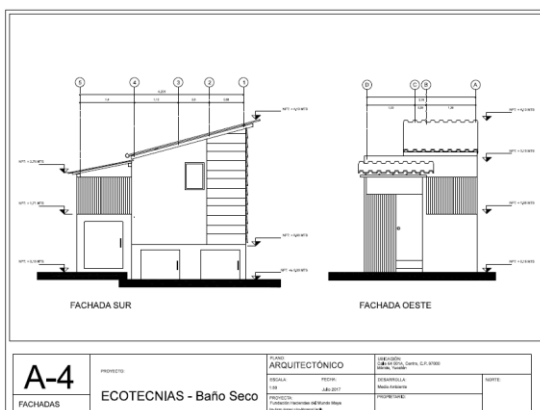
Planos de la fachada del baño seco. Veinte de Noviembre, Calakmul.
